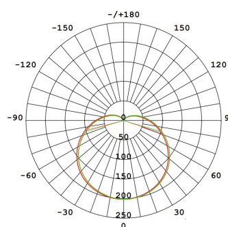
CURVA FOTOMETRICA
